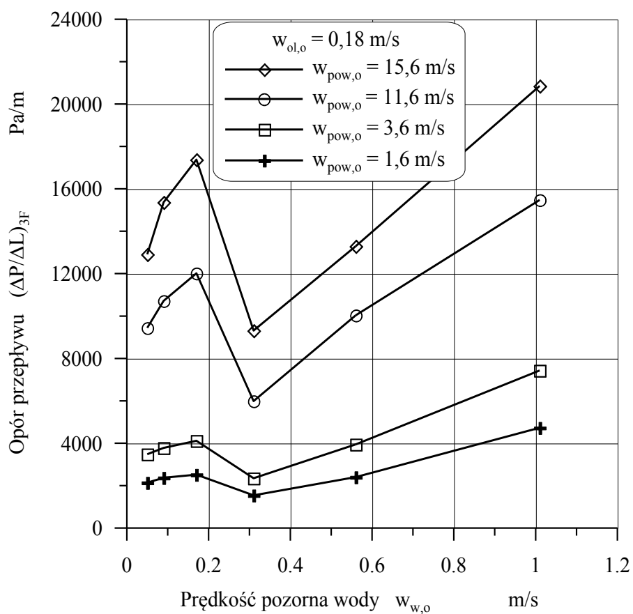
Rys. 5.3. Redukcja oporów przy przepływie trójfazowym przez kanał o średnicy 16 mm – wg [15]
